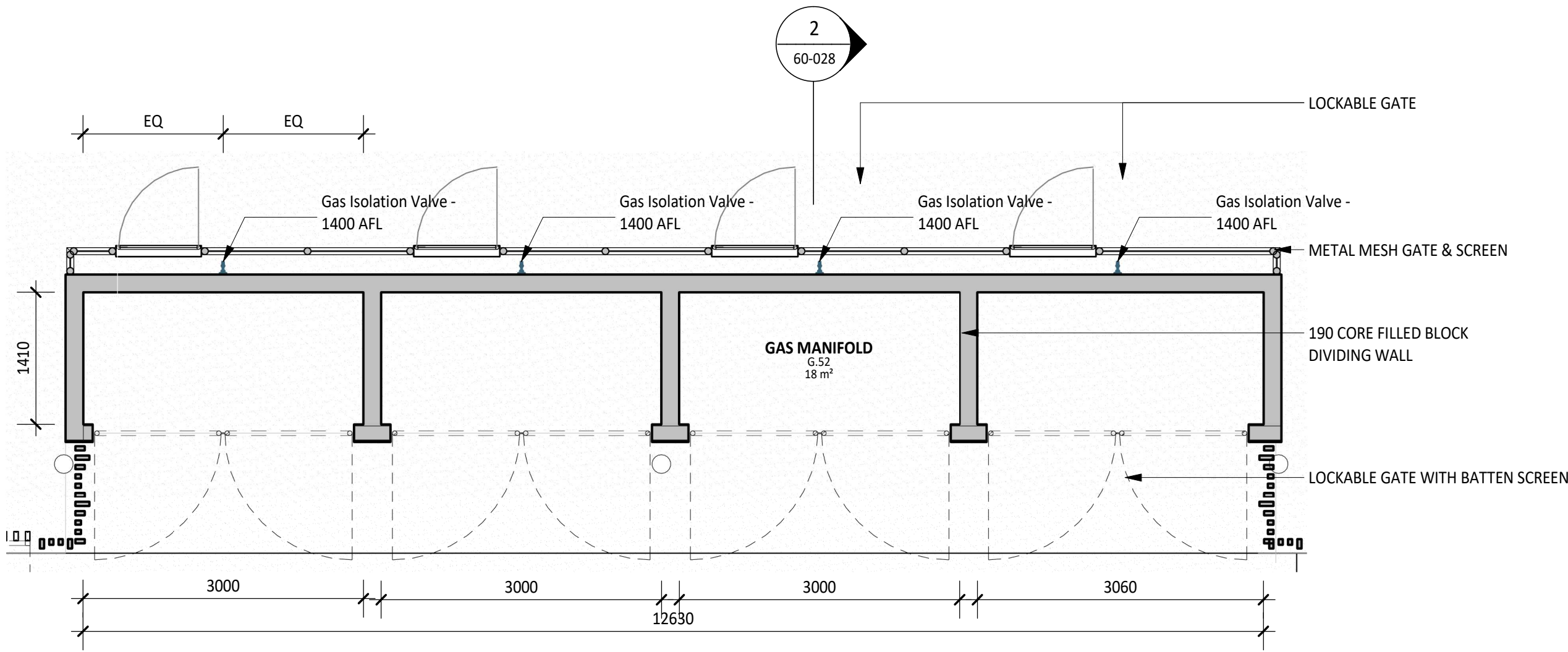
1 PLAN DETAIL 30-01 1 : 50
